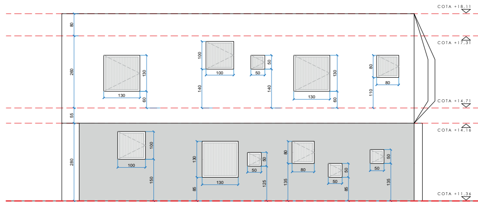
ALZADO ESTE
