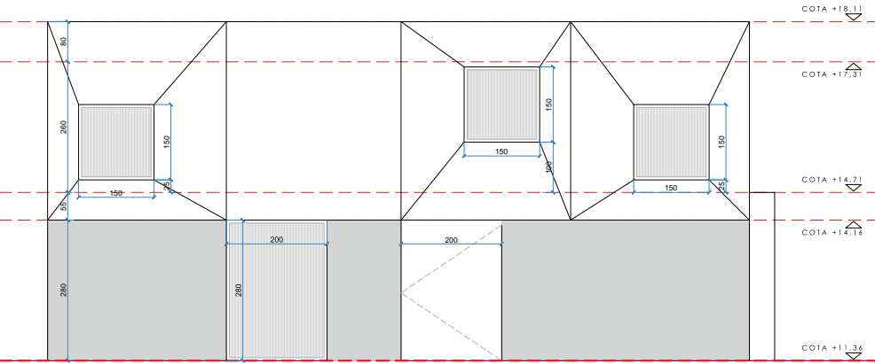
ALZADO NORTE
